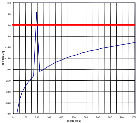
最大電圧（励振源電圧に対するプレーン上の最大値）
